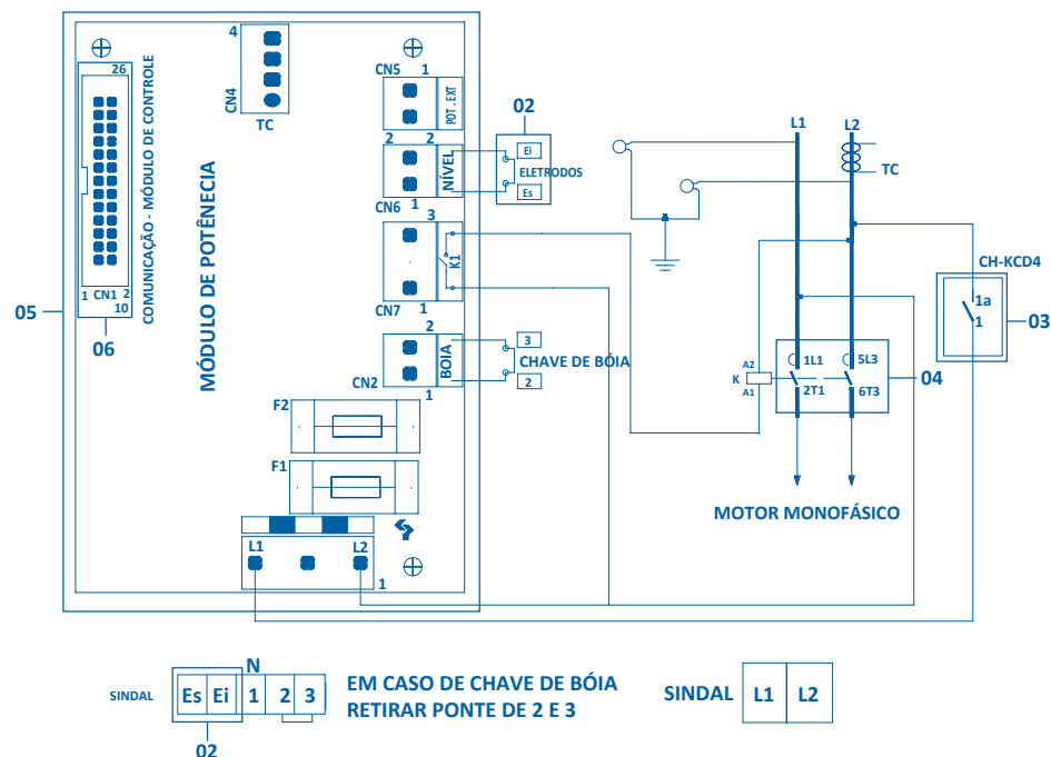
ESQUEMA ELÉTRICO MONOFÁSICO - SMART QC 0.5 A 5.5cv 220V M
