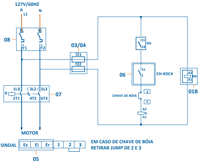
ESQUEMA ELÉTRICO MONOFÁSICO MDS - 1/2 A 1CV M - 127V
