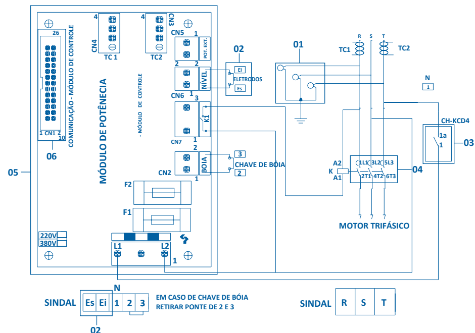
ESQUEMA ELÉTRICO TRIFÁSICO - SMART QC 0.5 A 7.5cv 380V T
