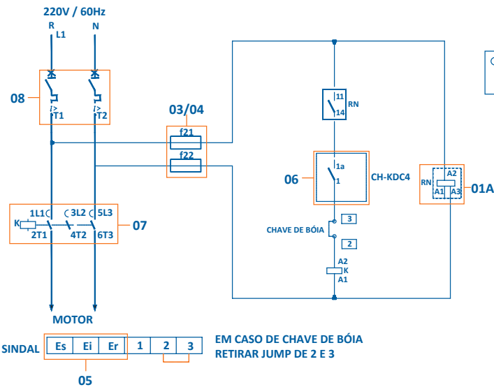
ESQUEMA ELÉTRICO MONOFÁSICO MDS - 1/2 A 5.1/2CV - 220V M
