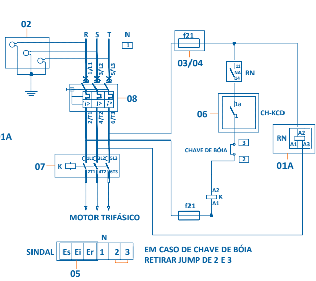
ESQUEMA ELÉTRICO TRIFÁSICO - 0.5 A 7.0CV
